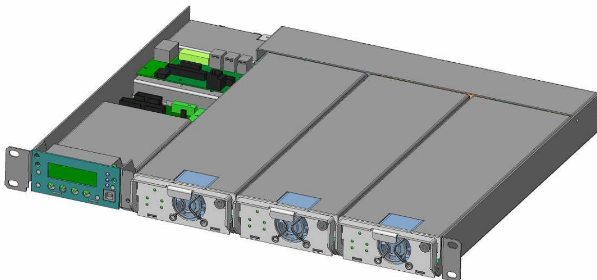
Рисунок 1.1 - Модульный каркас PS500KM с инверторами PS48-60/500К и контроллером Штиль PSC-200
