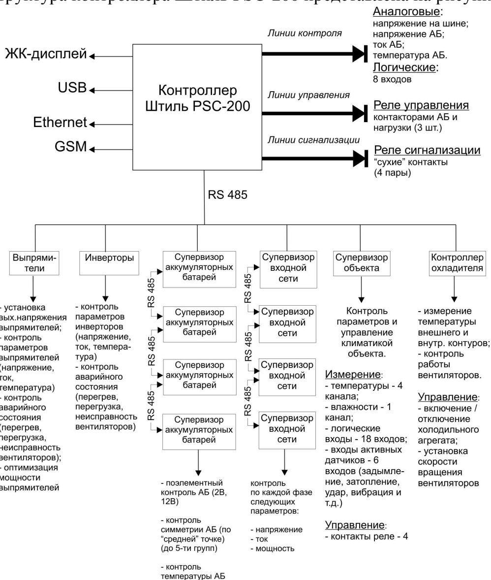
Рисунок 1.2 - Структура контроллера Штиль PSC-200 (максимальная конфигурация)
